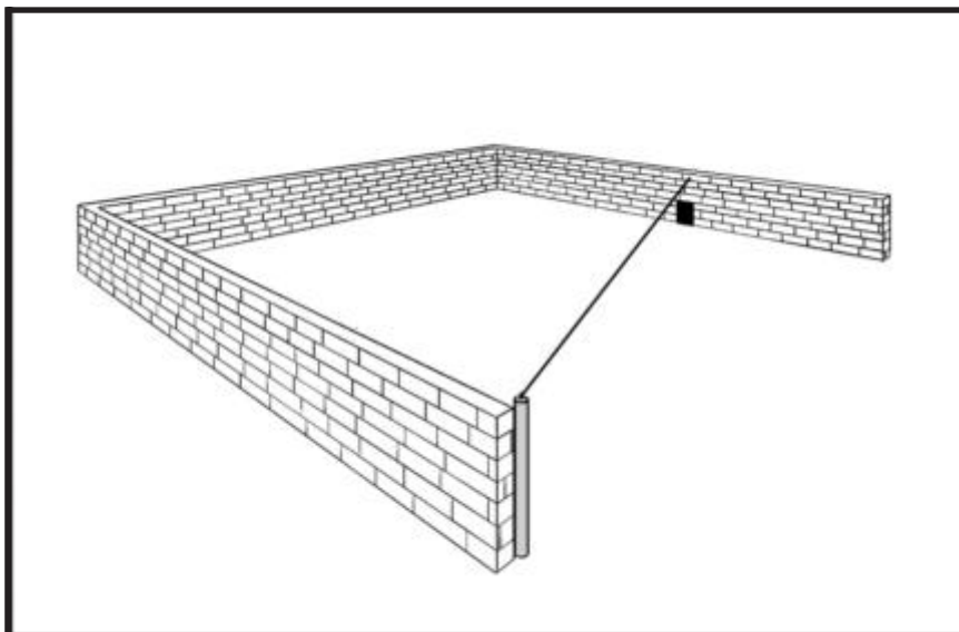
ציור ה - התקנת לחי מתחת לקנה העליון המחובר לדופן של אמצע הכותל
