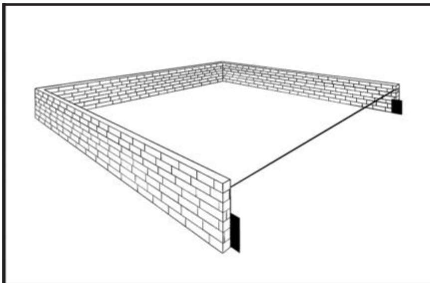
ציור ג - התקנת לחיים מתחת לקנה העליון המחובר לדופן של ראש הכותל משני צדדיו
