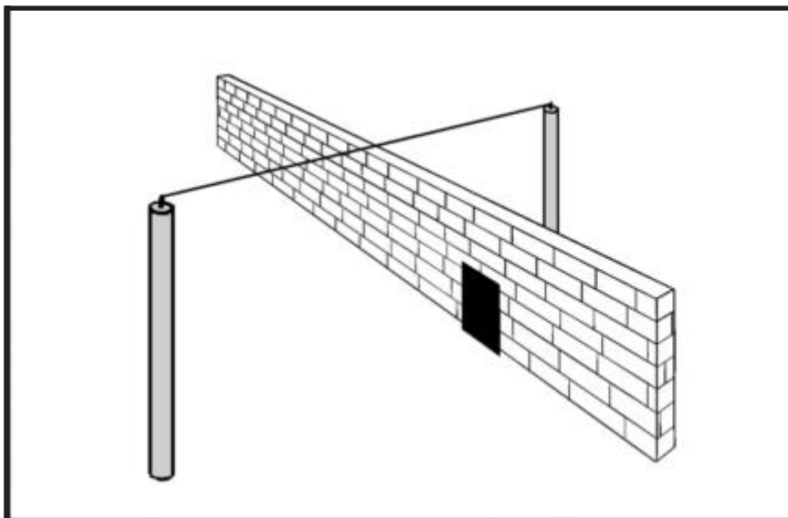
ציור ז - התקנת לחי בצורת הפתח הבנויה אחרי הכותל
