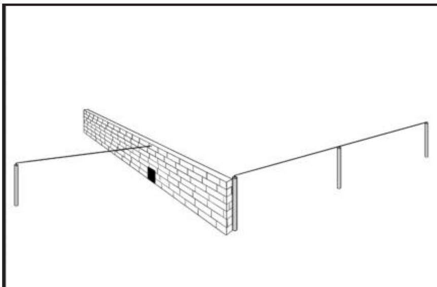
ציור ו - התקנת לחי מתחת לקנה העליון המחובר לדופן של אמצע הכותל
