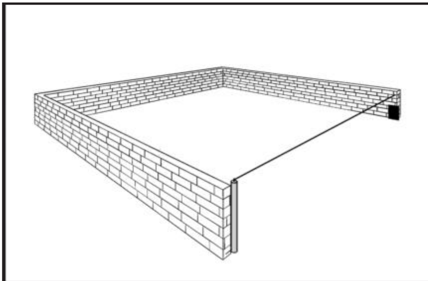
ציור ד - התקנת לחי מתחת לקנה העליון המחובר לדופן של ראש הכותל מצד אחד
